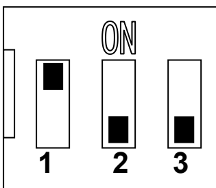
图 6 5# 模块地址
