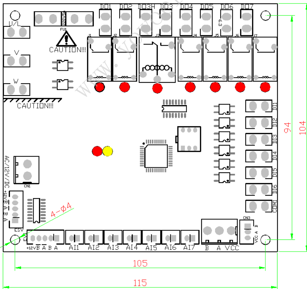
3、IO 板外形安装尺寸图
