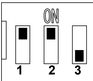
图 6 5# 模块地址
