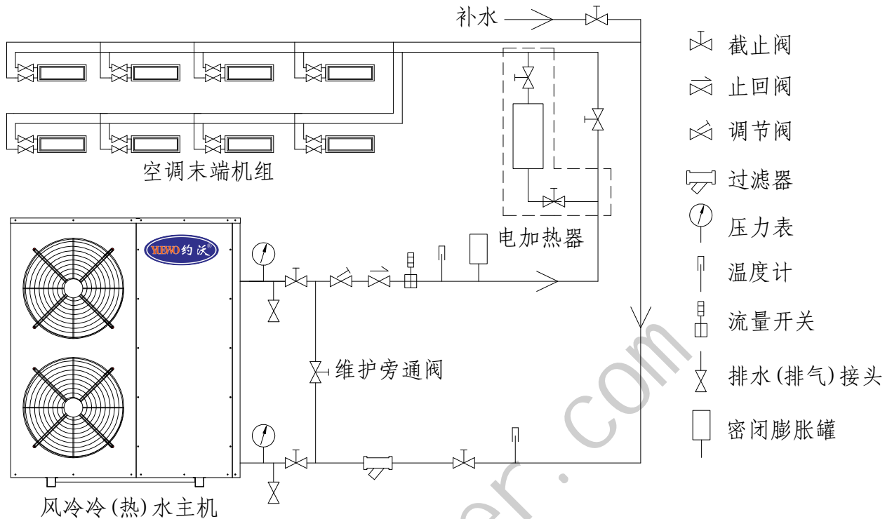
闭式水系统安装参考图
